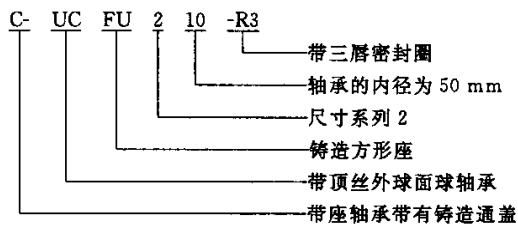
示例 2: 带有铸造盖并带铸造方形座顶丝外球面球轴承
