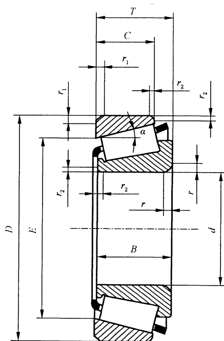
图 1 圆锥滚子轴承 30000 型
