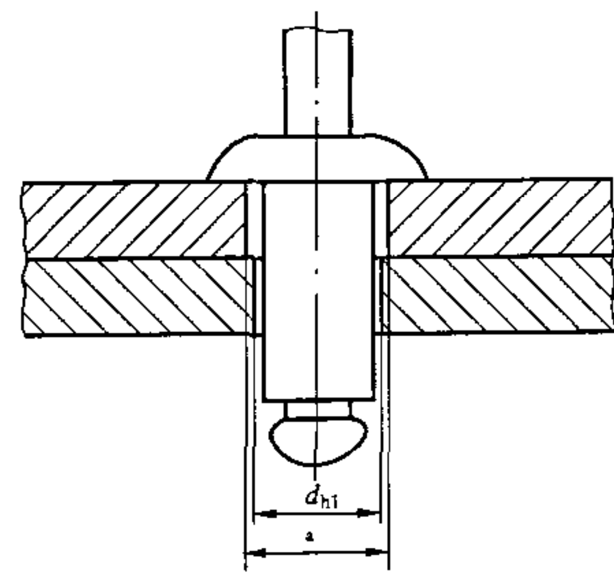
图 2 为便于对中加大的铆钉孔
