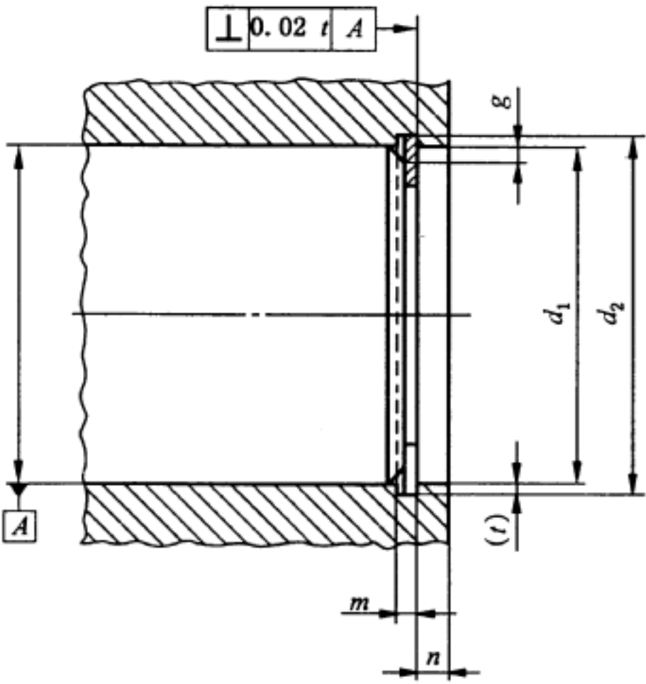
图 2 安装示例
