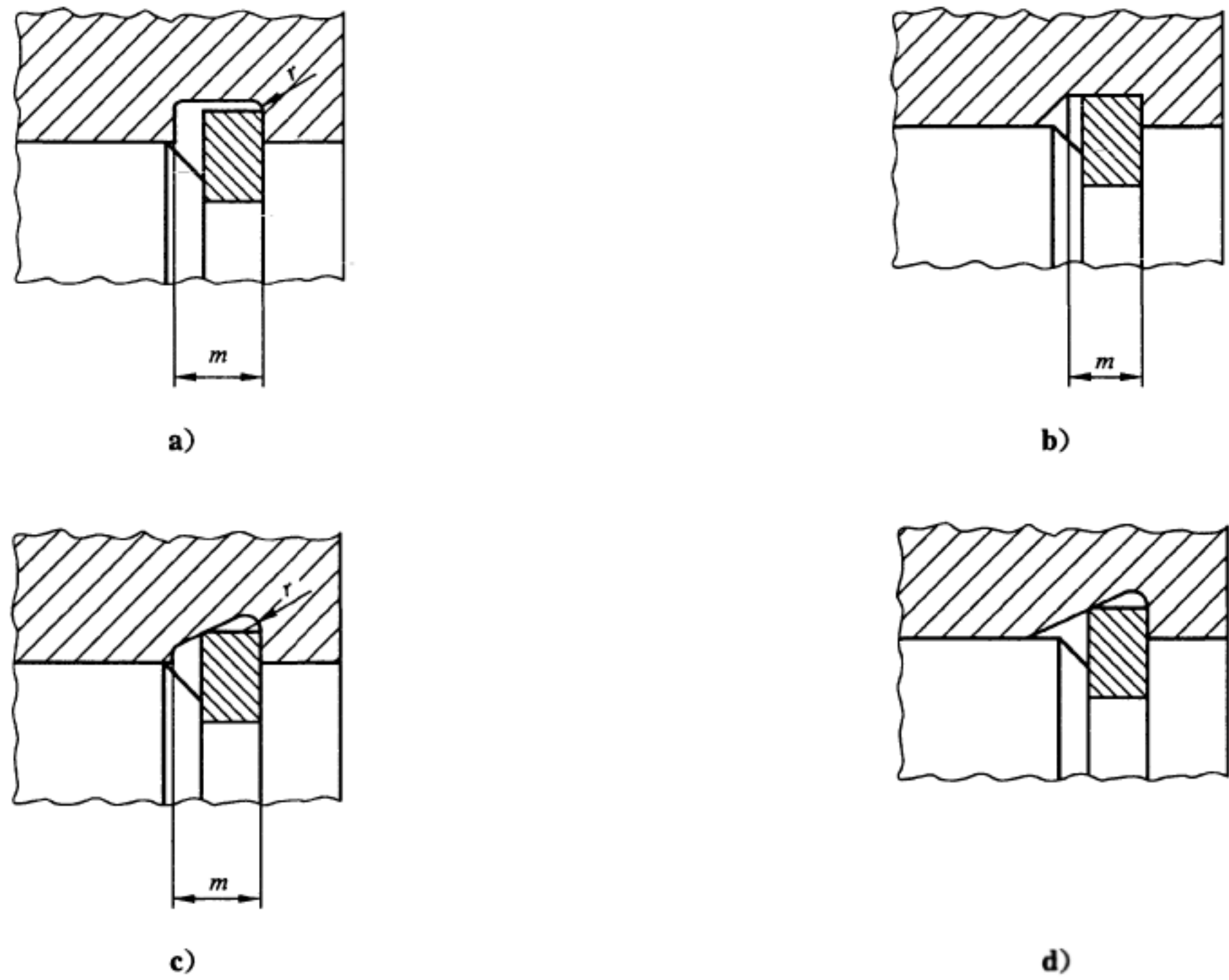
图 6 沟槽形状
