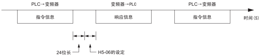
图 C.8 响应等待时间
