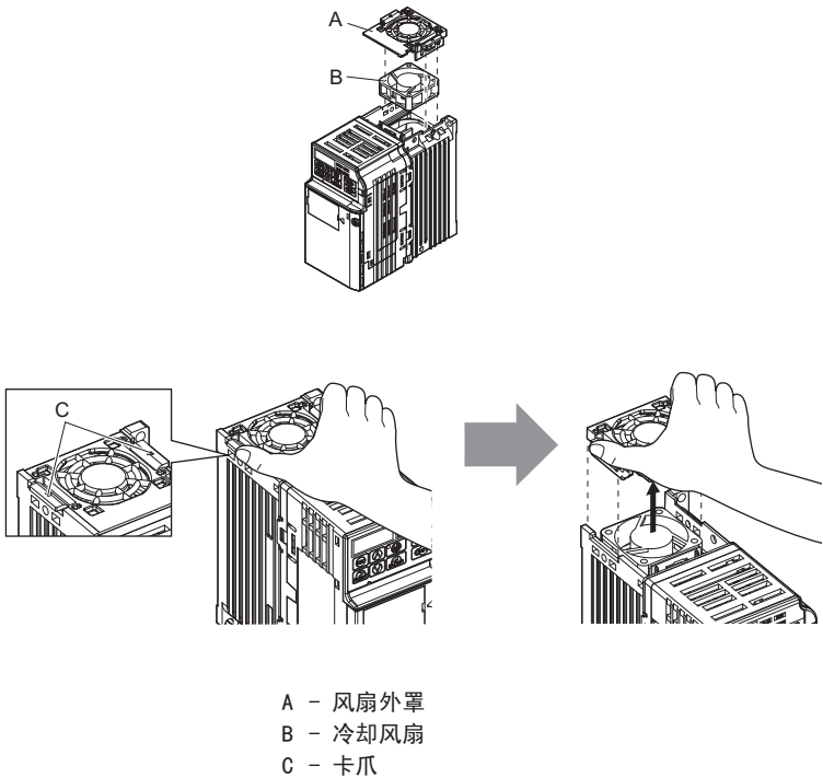
图 7.1 风扇外罩的拆卸
