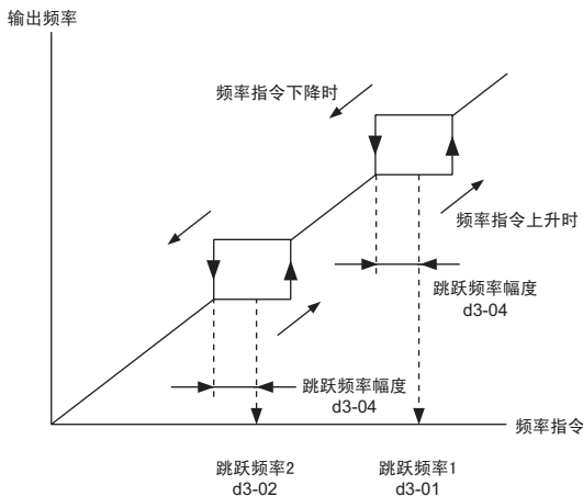
图 5.9 跳跃频率
