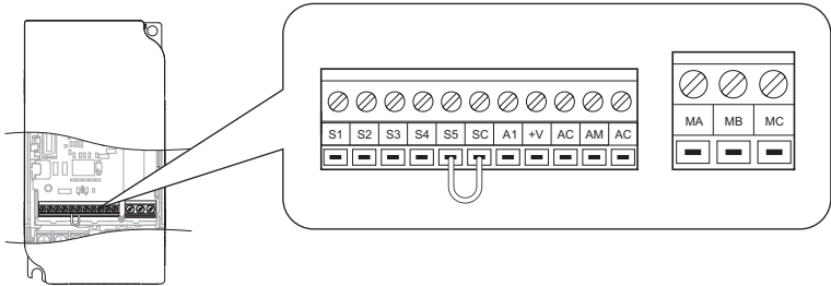
图 C. 11 执行自检时变频器端子的连接
