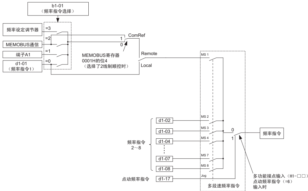
图 5.6 频率指令部框图
