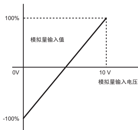
图 5.24 无 0 极限的模拟量输入 (偏置设定 -100%)
