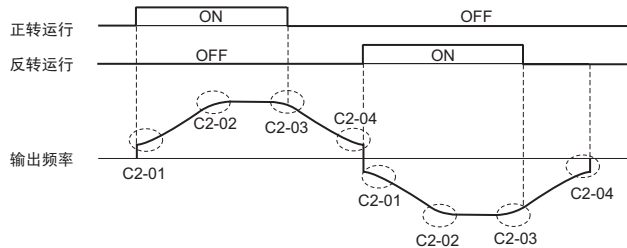
图 5.4 正转 / 反转切换时的 S 字特性
