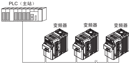
图 C.1 PLC 和变频器的连接例
