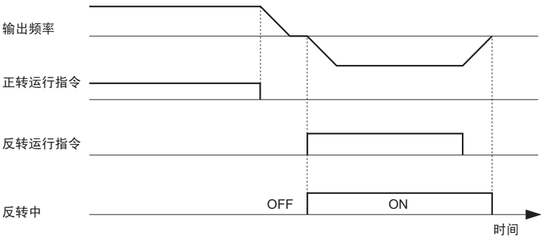
图 5.22 反转中输出时序图
