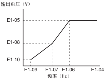
图 5.11 V/f 曲线图
