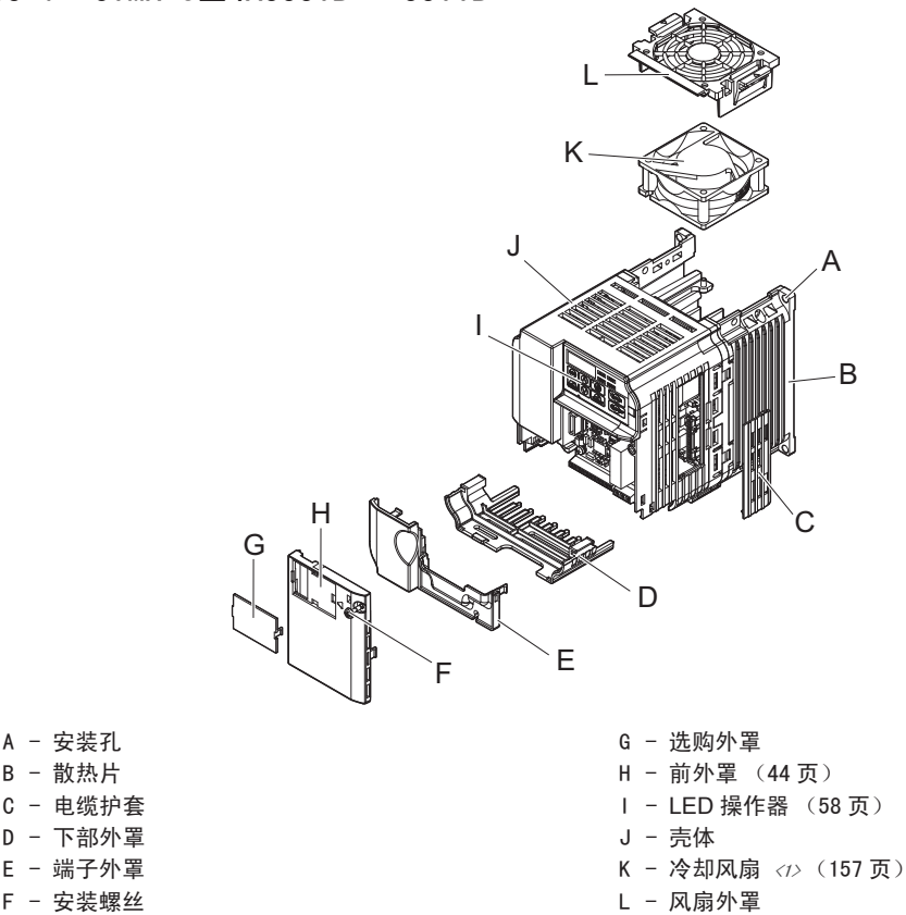
图 1.3 柜内安装型变频器各部分的名称 C1MR-J□2A00012B
