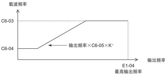
图 5.5 与输出频率相应的载波频率的变化
