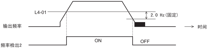
图 5.34 频率检出 2
