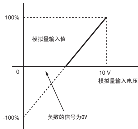
图 5.23 有 0 极限的模拟量输入 (偏置设定 -100%)
