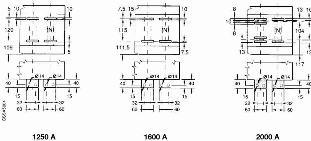
后水平端子
