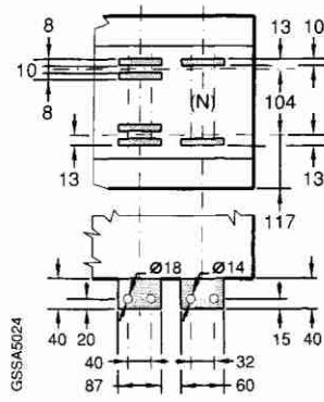
后水平端子
