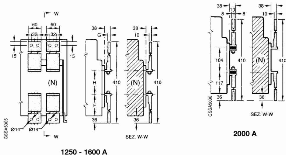
前接线端子
