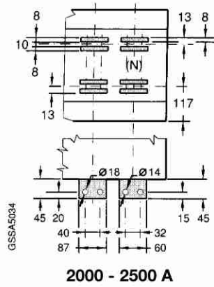
后水平端子
