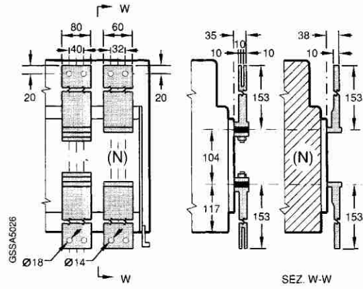
前接线端子
