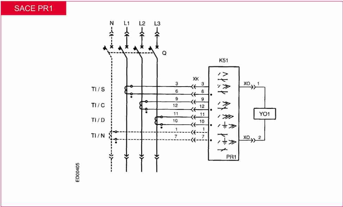
使用 SACE PR1 固态微处理器控制的脱扣器的 Megamax F 断路器
