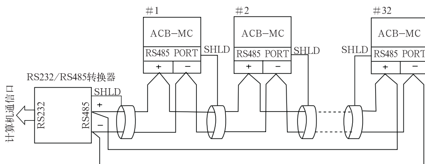
图9 ACB-MC通信的环形连接方式
