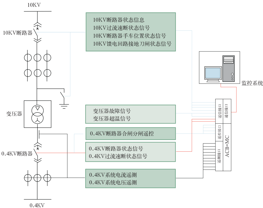
图7 ACB—MC在中低压回路的监视和告警示意图
