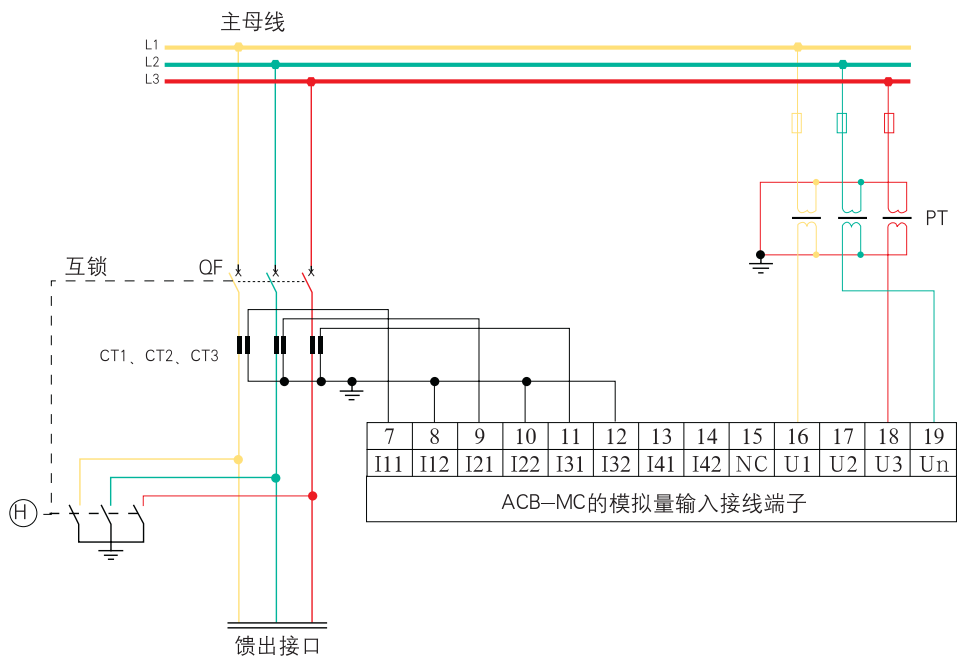
图5 在10KV下利用ACB-MC采集电流电压接线图
