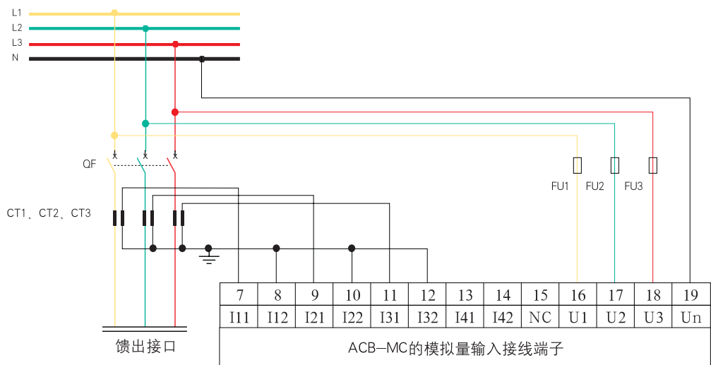
图4 在0.4KV下利用ACB-MC采集电压及电流接线图
