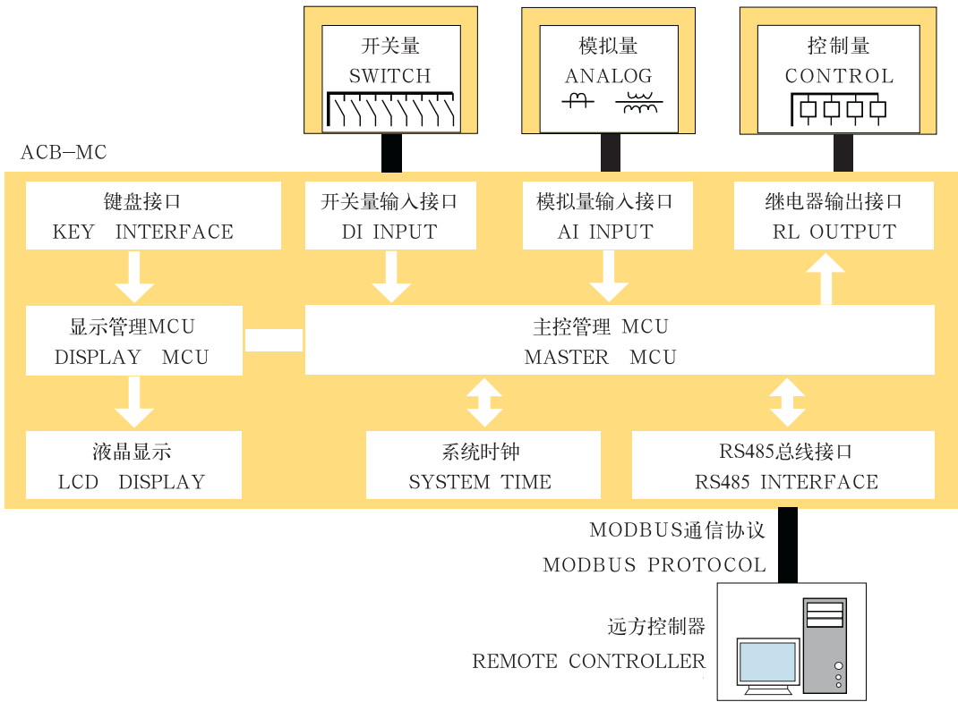
图2 ACB-MC结构框图和信息流程图
