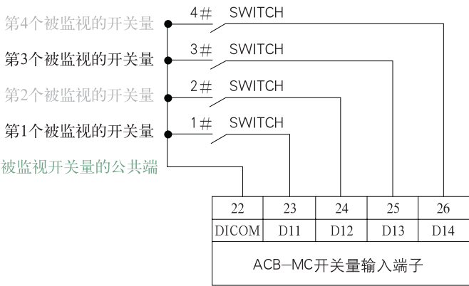
图6 遥信开关量监视接线图
