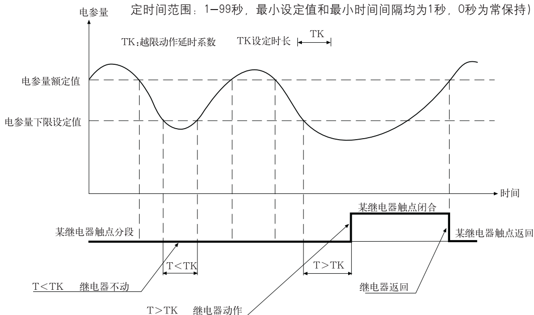
图10 ACB-MC继电器工作特性曲线
