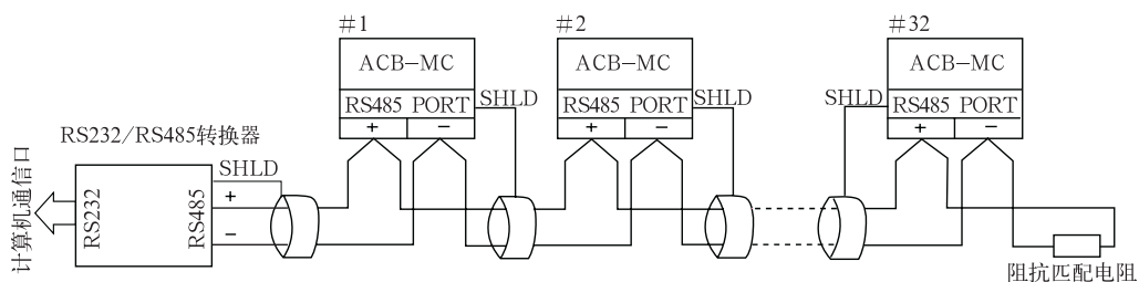
图8 ACB-MC通信的线形连接方式
