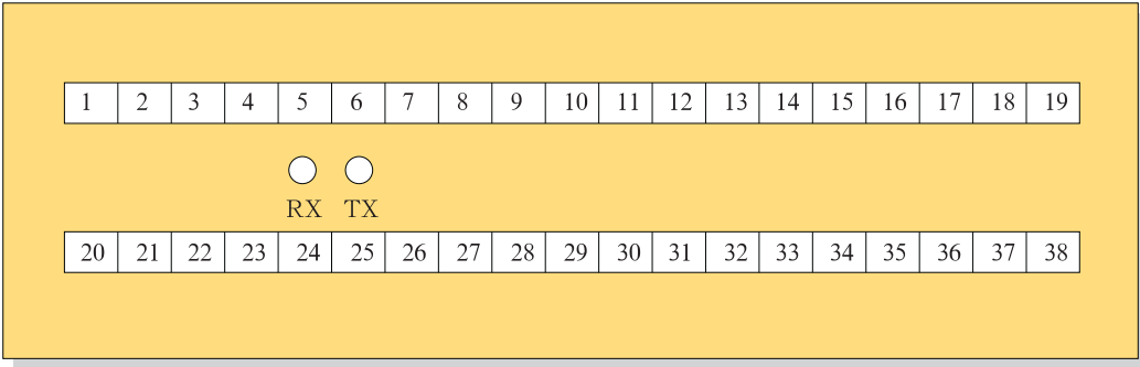
图3 ACB—MC接线端子图
