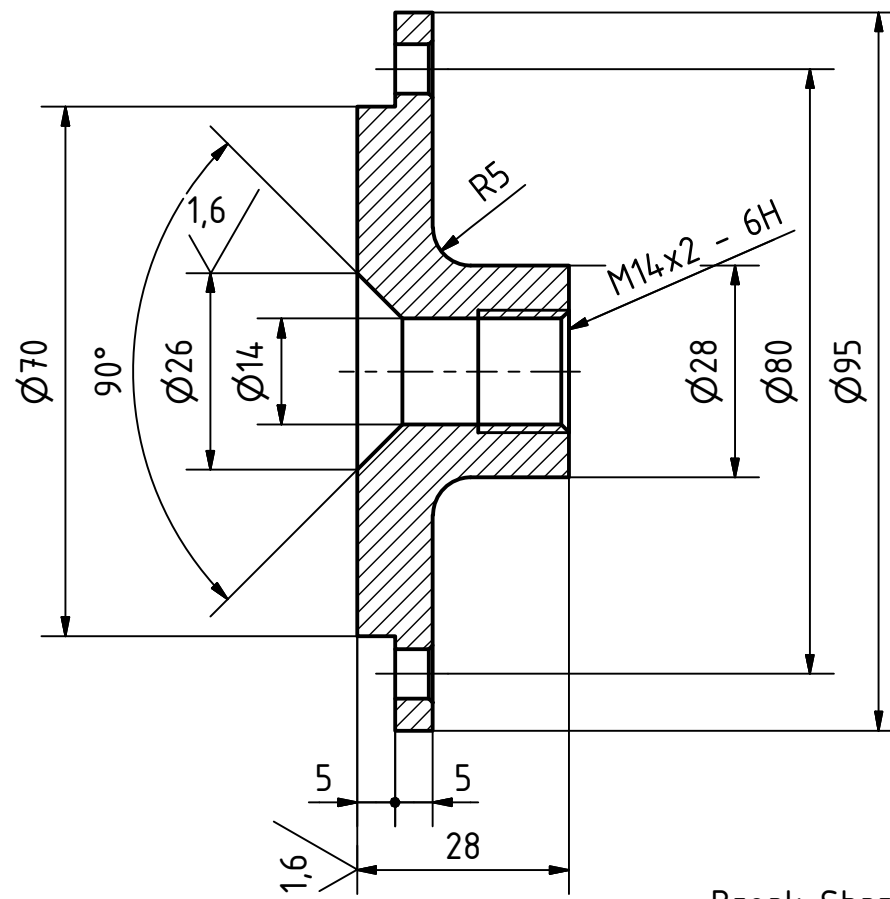
A-A ( 1 : 1 )
